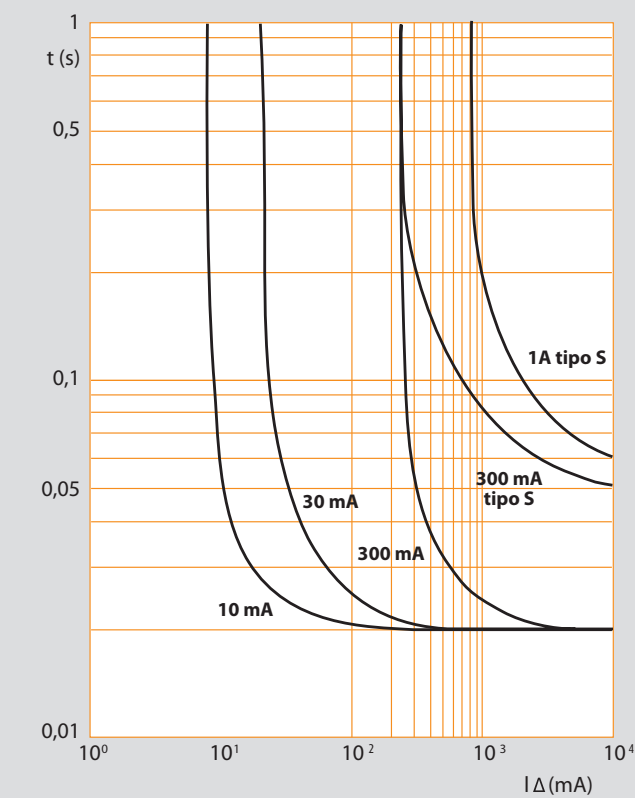
DIFERENCIAL PURO 2P - 4P
