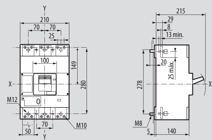
DIMENSIONES M5 1600N/H
