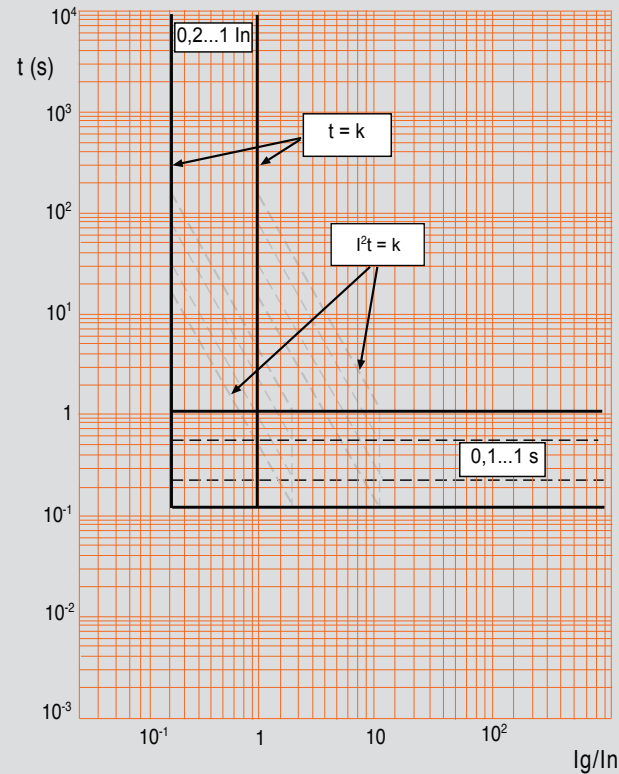
CURVA DE INTERVENCIÓN PARA FALLA A TIERRA (MP4 Y MP6 LSIg)
