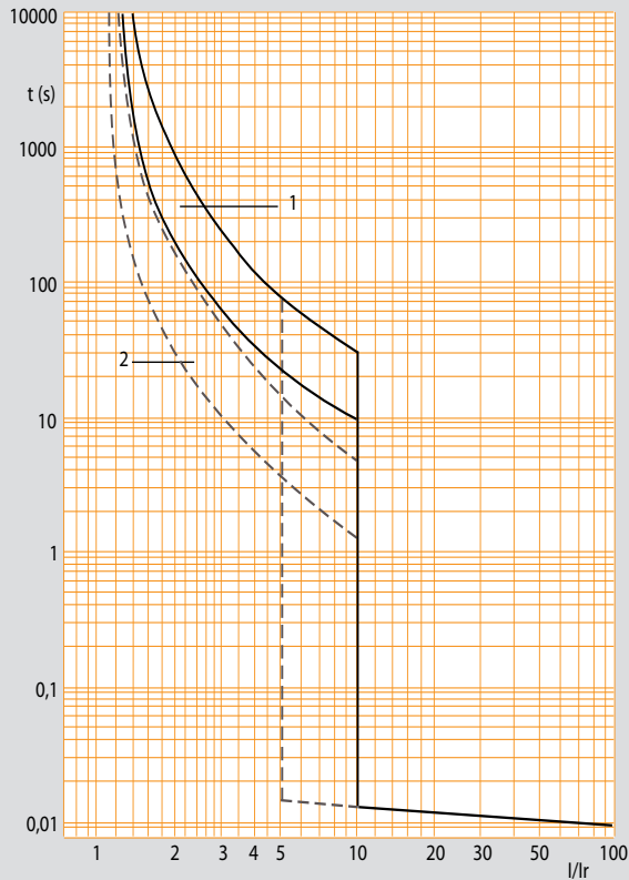
TIEMPO-CORRIENTE
