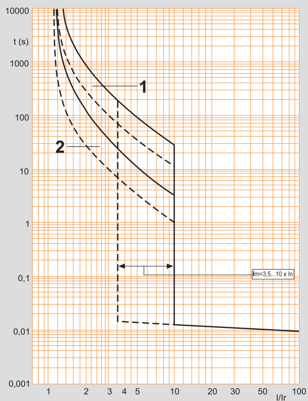
TIEMPO-CORRIENTE
