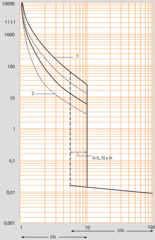
TIEMPO-CORRIENTE
