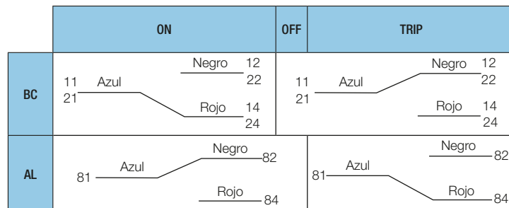
Diagrama de Conexión del Interruptor DWB1600
